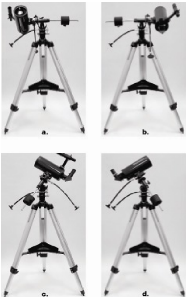
Рисунок 8. Здесь показан телескоп, ориентированный в четырех направлениях: (а) север, (b) юг, (с) восток, (d) запад. Обратите внимание, что тренога и штатив не должны перемещаться; только труба телескопа должна поворачиваться вокруг осей склонения и восхождения.
