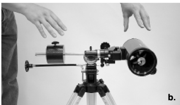
Рисунок 4. Для правильного ориентирования телескопа необходимо сбалансировать трубу на оси прямого восхождения (а). Передвиньте противовес так, чтобы он уравновешивал трубу
